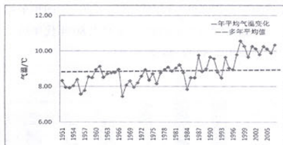
图 2-1 银川年平均气温变化曲线
