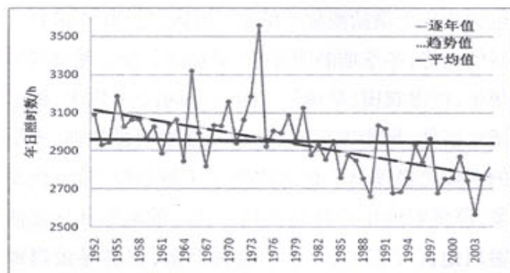
图 2-5 银川市年日照时数逐年值和气候趋势值变化图
