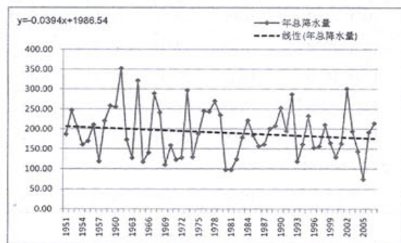
图 2-3 1951-2007 年年总降水量变化趋势
