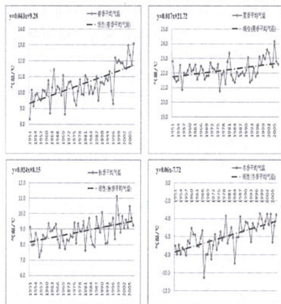
图 2-2 银川各季平均温度变化趋势图
