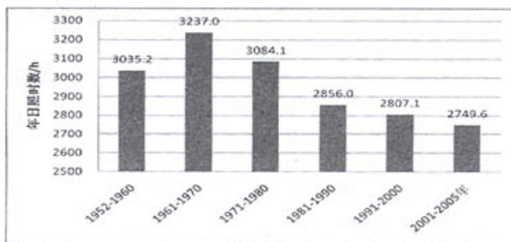
图 2-5 银川市各年代年均日照时数
